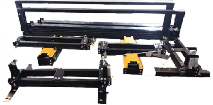
MRL 2:1 CARFRAME
