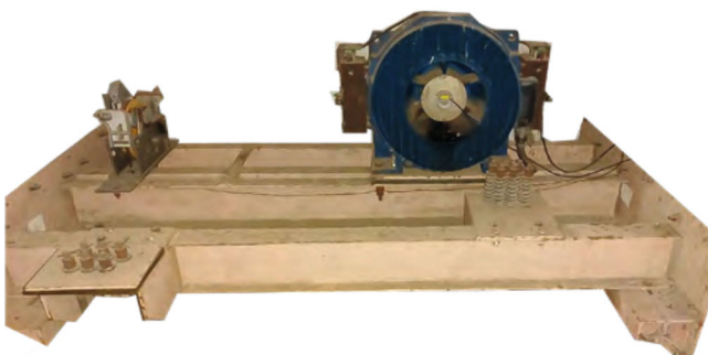
MINI MACHINE ROOM
